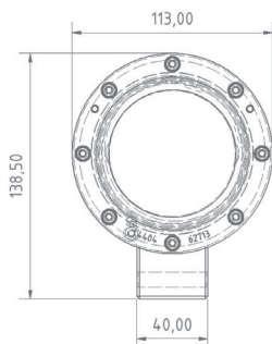
T08-VA2.1.X.X Vorderansicht
