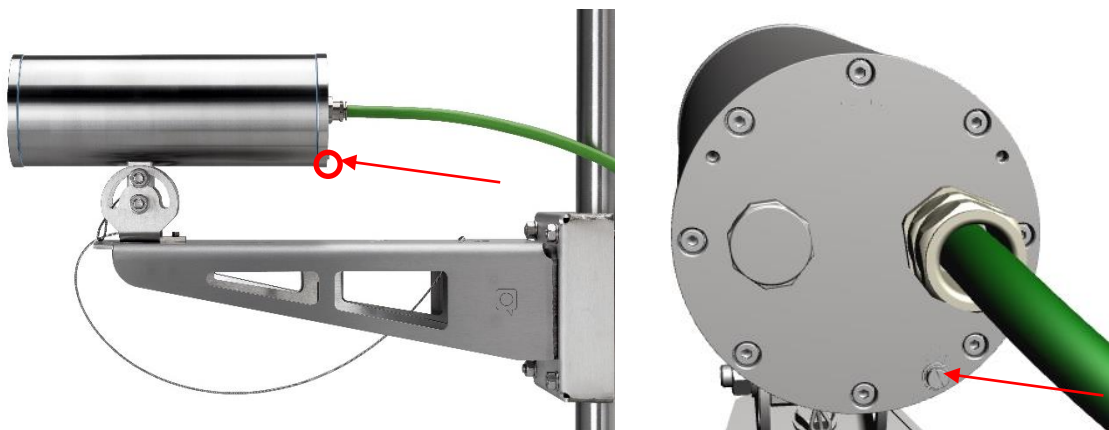
Bild 5-1 ExCam IPQ1615 Potentialausgleich
