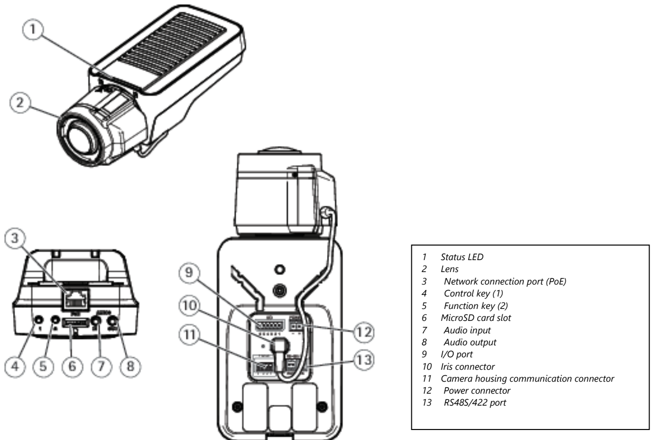
Bild 6-4 Aufbau der Kamera (Abb. ähnlich)
