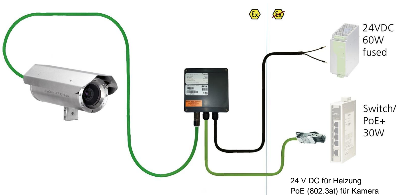
Bild 5-9 ExTB-3 -> Sicherer Bereich
