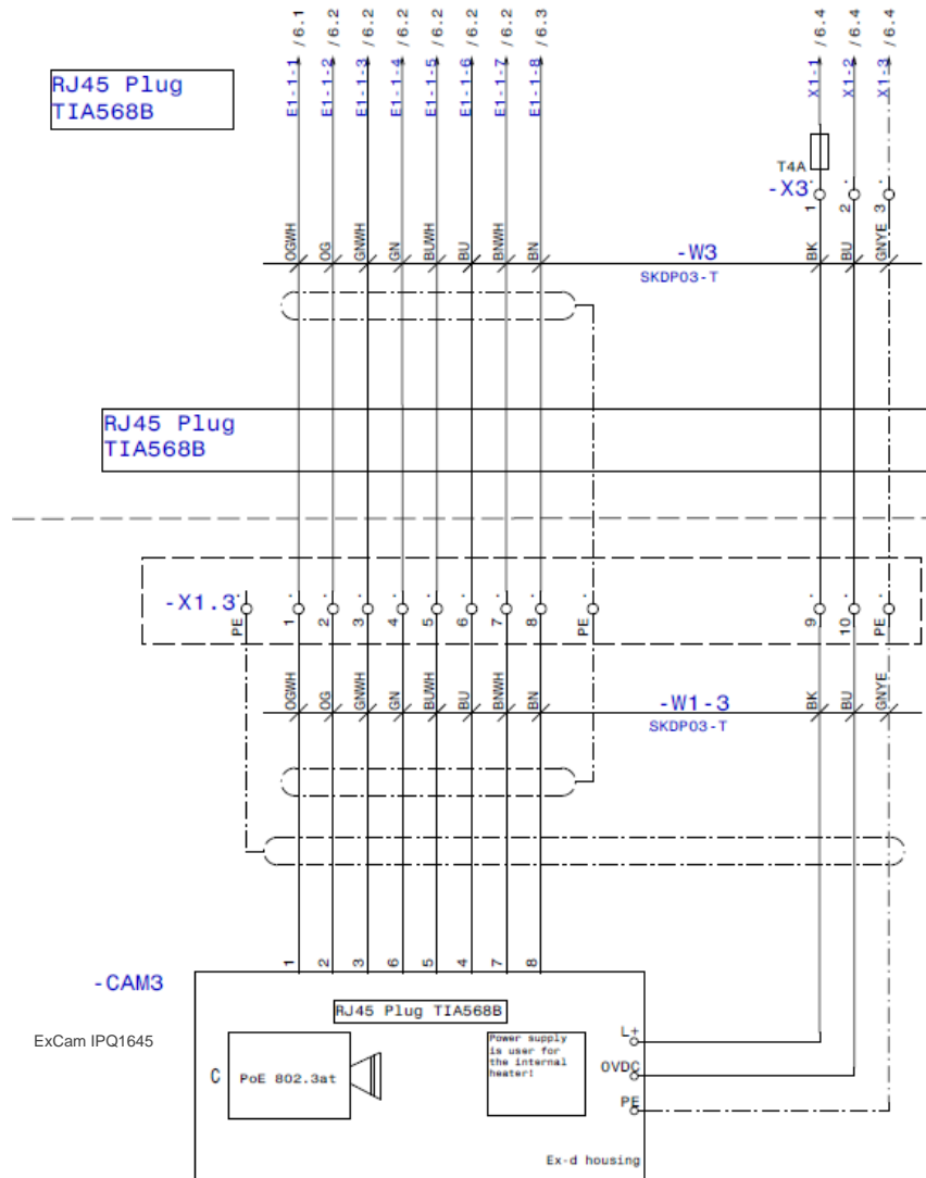
Bild 5-7 Musterbeschaltung des Klemmkastens ExtB-3 (mit Heizung)
