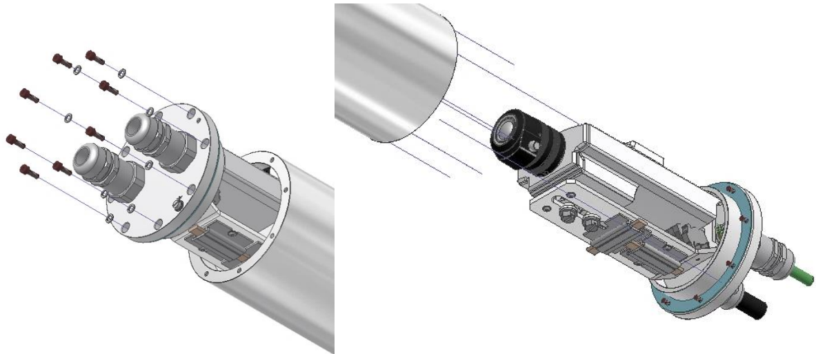
Bild 6-3 Öffnen der ExCam IPQ1615 (Abb. ähnlich)
