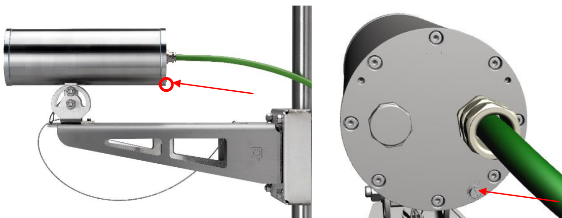
Bild 5-1 ExCam IPQ1645 Potentialausgleich
