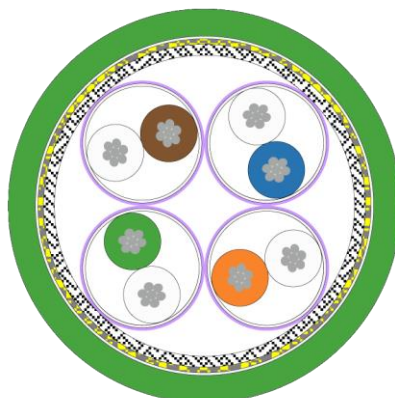
Bild 2-5 Schnittdarstellung SKD05-HT
