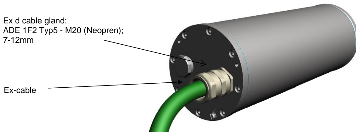
Bild 5.2 – Ex d Kabelverschraubung und Zuleitung
