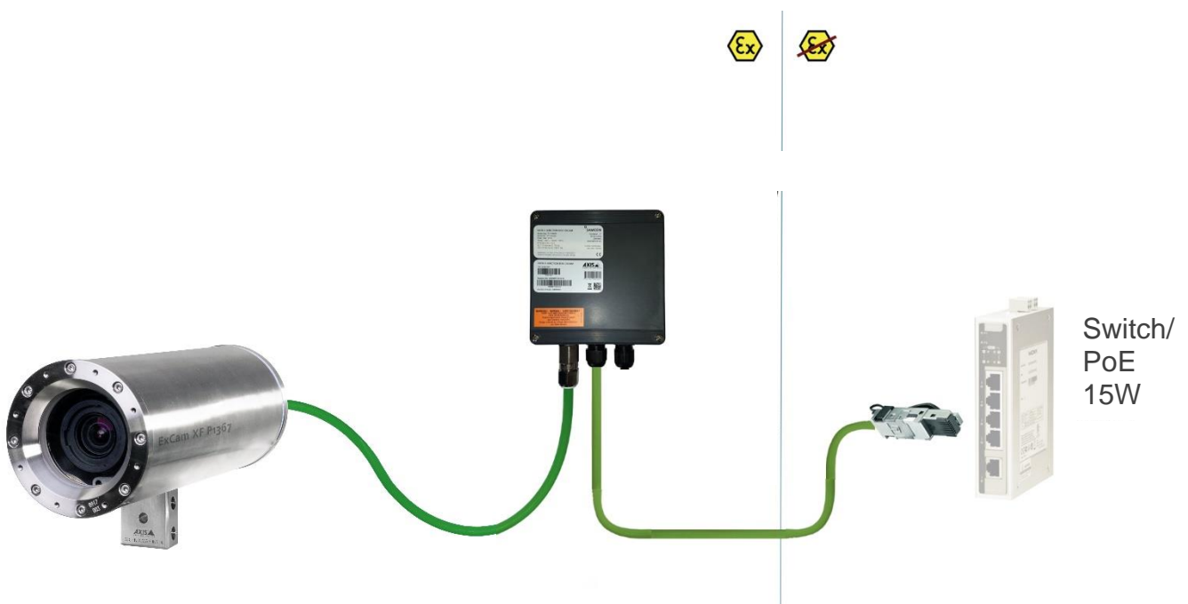
Bild 5-6 ExTB-3 -> Sicherer Bereich
