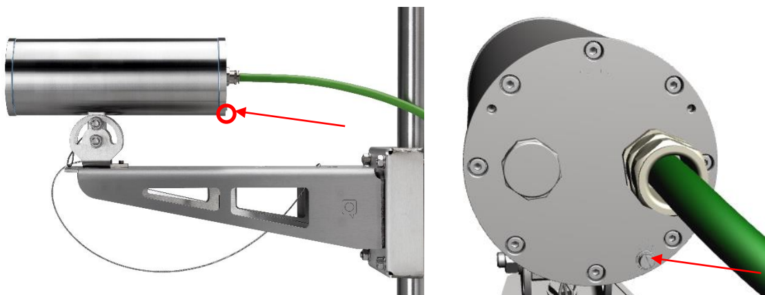
Bild 5-1 RoughCam IPP1377 Potentialausgleich
