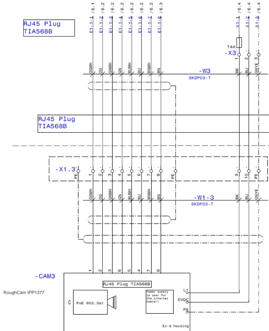
Bild 5-7 Musterbeschriftung des Klemmkastens ExtB-3 (mit Heizung)
