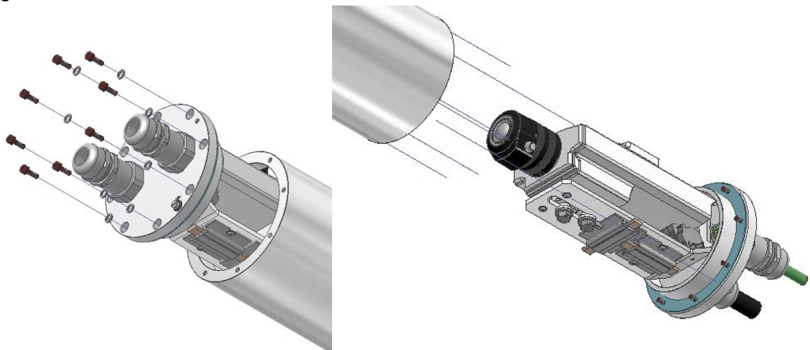
Bild 6-3 Öffnen der RoughCam IPP1377 (Abb. ähnlich)
